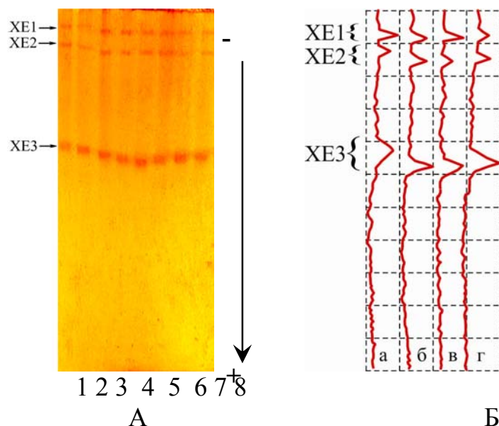
Рис 2. Ізоферменти холінестерази тканин репродуктивних органів бугаїв; А — копії фореграм ХЕ: 1, 2 — сім'яника; придатка: 3, 4 — голівки; 5, 6 — тіла; 7, 8 — хвоста; Б — денситограма білків холінестерази; а — сім'яник; придаток сім'яника: б — голівка; в — тіло; г — хвіст; ХЕ1–ХЕ3 — ізоформи ферменту
